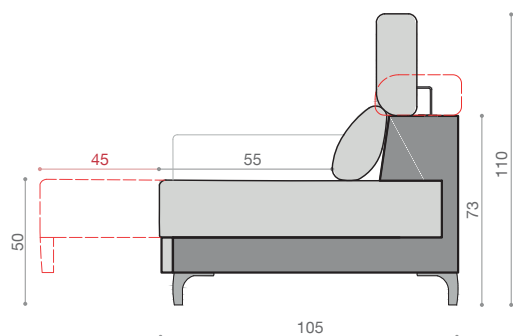
SECCIÓN MÓDULO SOFÁ SECTION MODULE CANAPÉ
